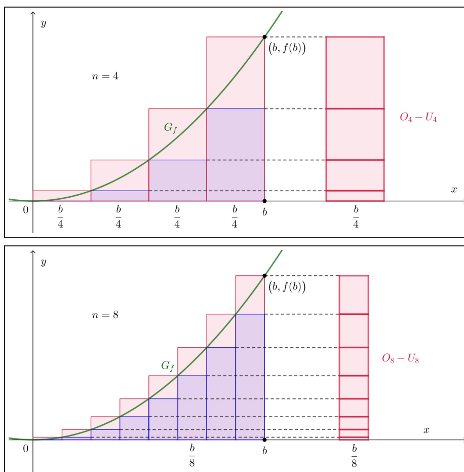
Abbildung 2.2: Der Differenz von Ober- und Untersumme entspricht einfach zu berechnende Fläche.
