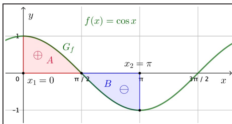
Abbildung 1.3: Das Integral von 0 bis \pi ergibt 0, weil A und B gleich gross sind, im Integral aber verschiedene Vorzeichen erhalten. Um A + B zu berechnen, müssen die Teilflächen daher separat bestimmt werden.
